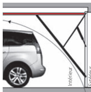
Cinématique porte DL-IL
