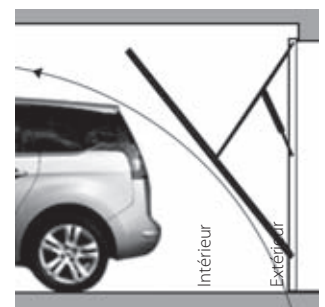
Cinématique porte OD-IL
